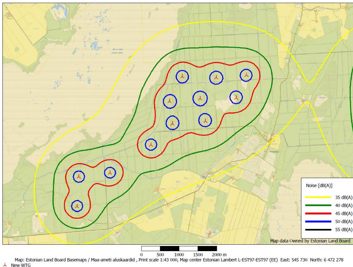
Joonis 21. Illustreeriv mürakaart ala 1 puhul.
