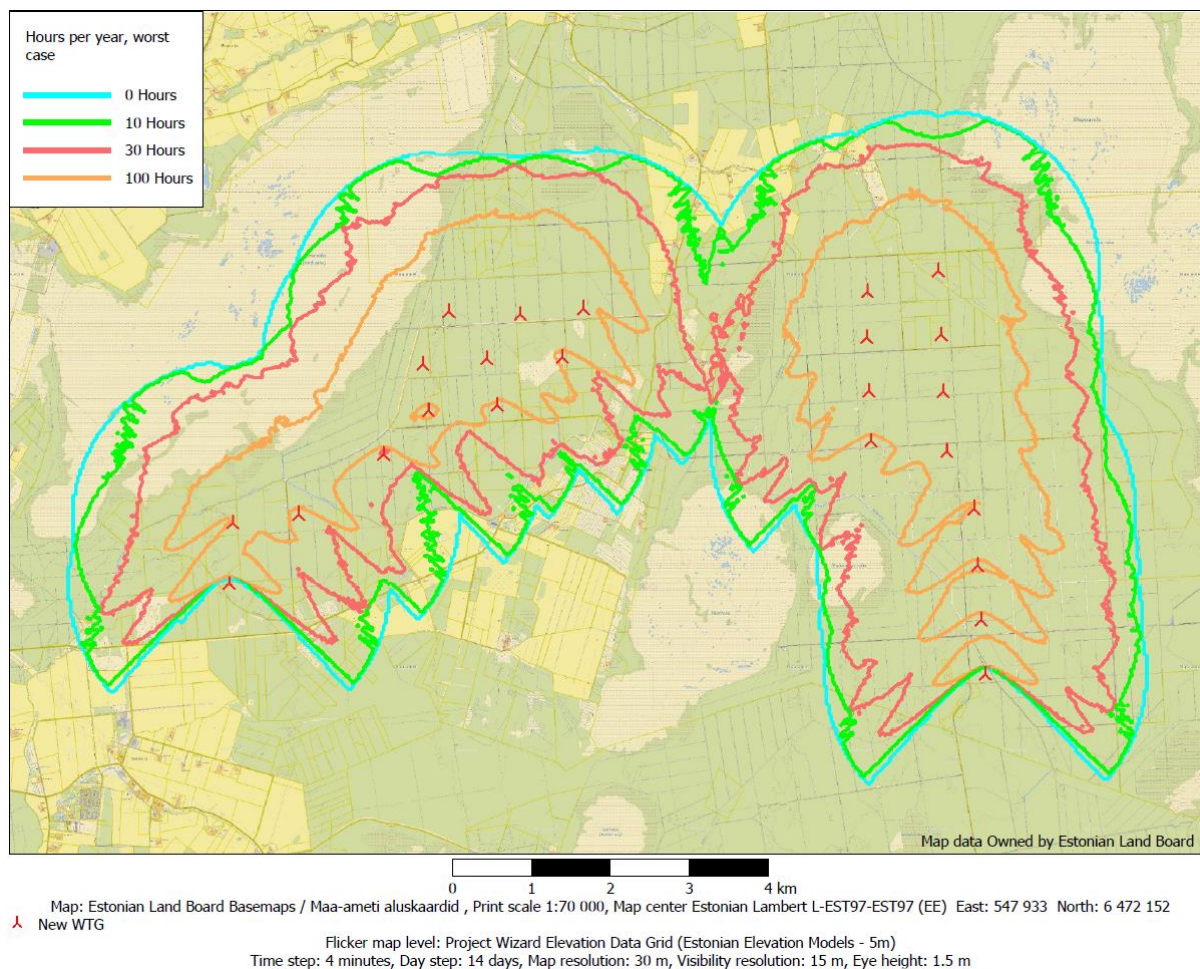
Joonis 23. Illustreeriv varjutuskaart halvim olukord (nn worst case ) ilma päikesepaiste kestvust arvestamata 290 m tipukõrgusega tuulikute korral. Kuna ala 1 ja ala 2 puhul oleks varjutusest mõjutatud erinevad elamualad, siis on varjutuskaart esitatud aladel ühiselt. Joonis illustreerib pigem varjude maksimaalset ulatust.
