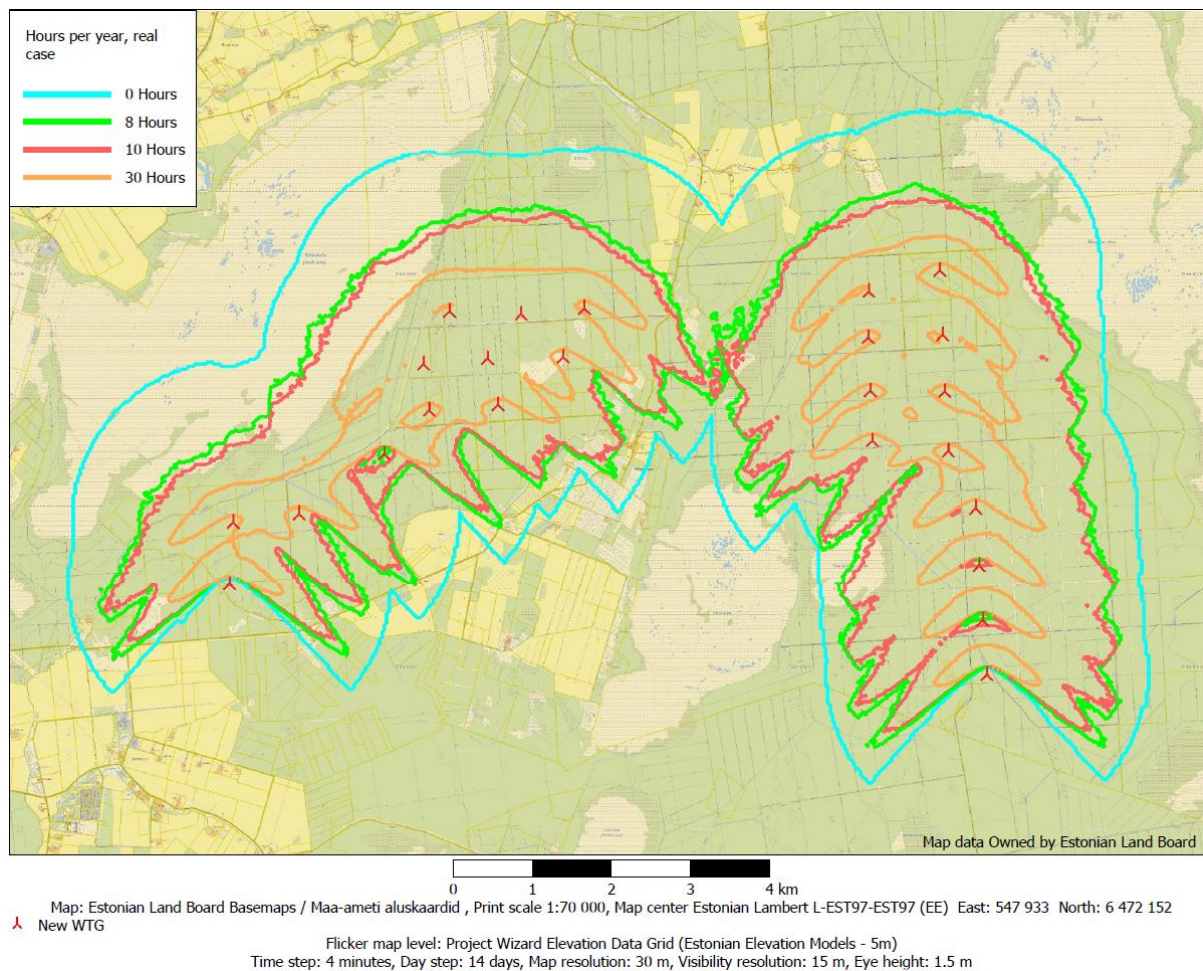
Joonis 24. Illustreeriv varjutuskaart reaalse olukord ilma kõrghaljastust arvestamata 290 m tipukõrgusega tuulikute korral. Kuna ala 1 ja ala 2 puhul oleks varjutusest mõjutatud erinevad elamualad, siis on varjutuskaart esitatud aladel ühiselt.
