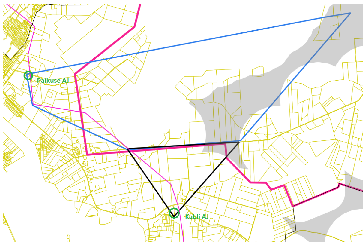
Joonis 41. Põhivõrguga liitumise alternatiivsed ühendused.
