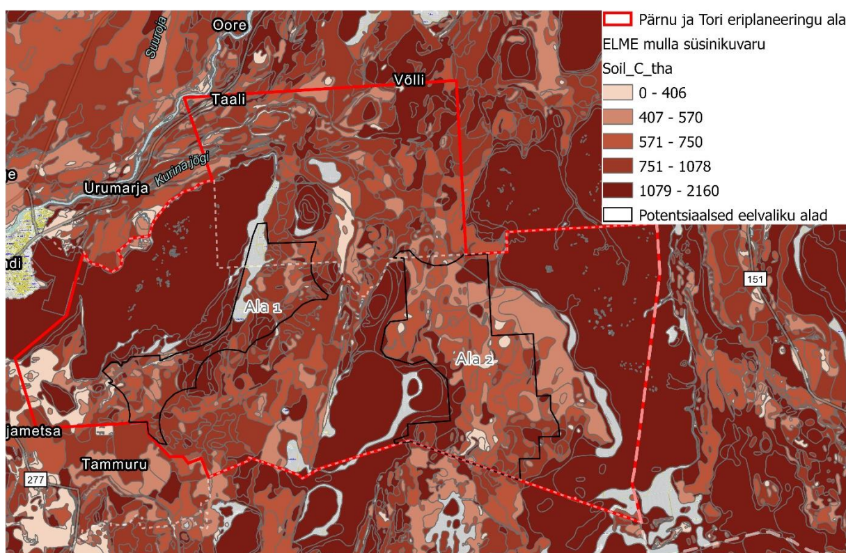
Joonis 38. Süsinikuvaru mullas. Alus: Keskkonnaagentuur ELME projekt.
